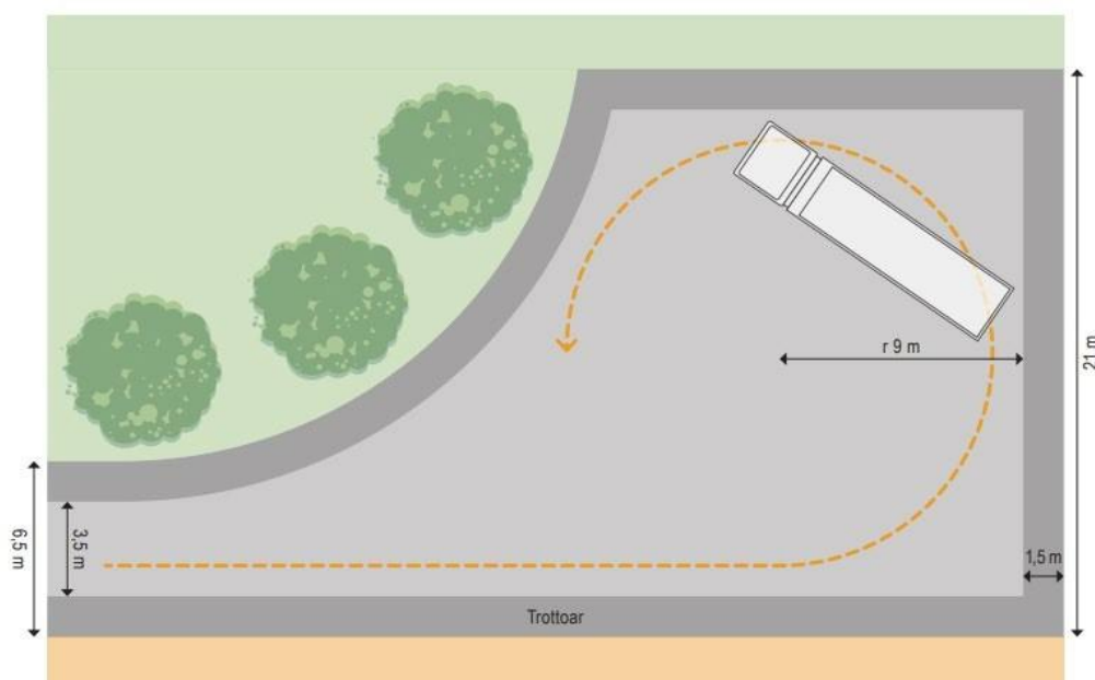
Figur 2 Alternativ vändplats till figur 1, för baklastande hämtningsfordon.
