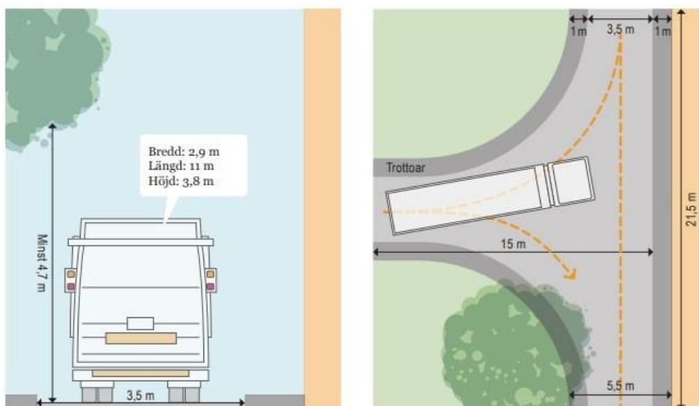
Figur 1 Vändplats för baklastande hämtningsfordon.
