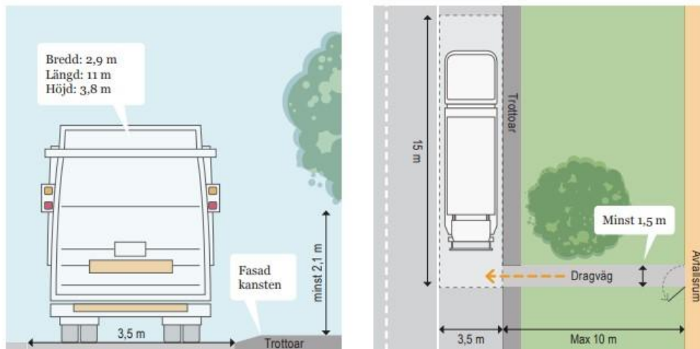
Figur 3 Dragväg och baklastare.
