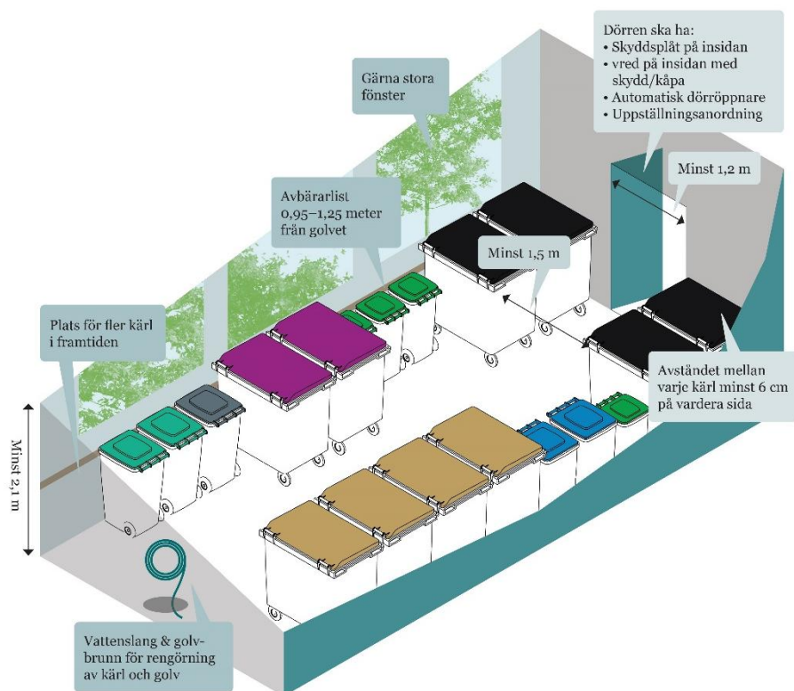
Figur 6 Exempel på avfallsutrymme med utbyggd fastighetsnära insamling.
