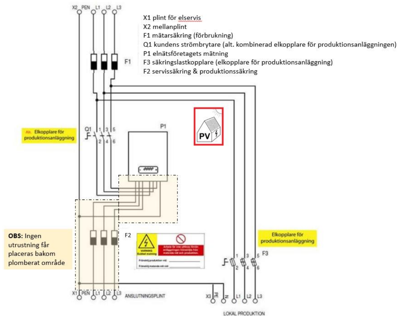
Figur 8 Inkoppling och märkning – produktionssäkring
