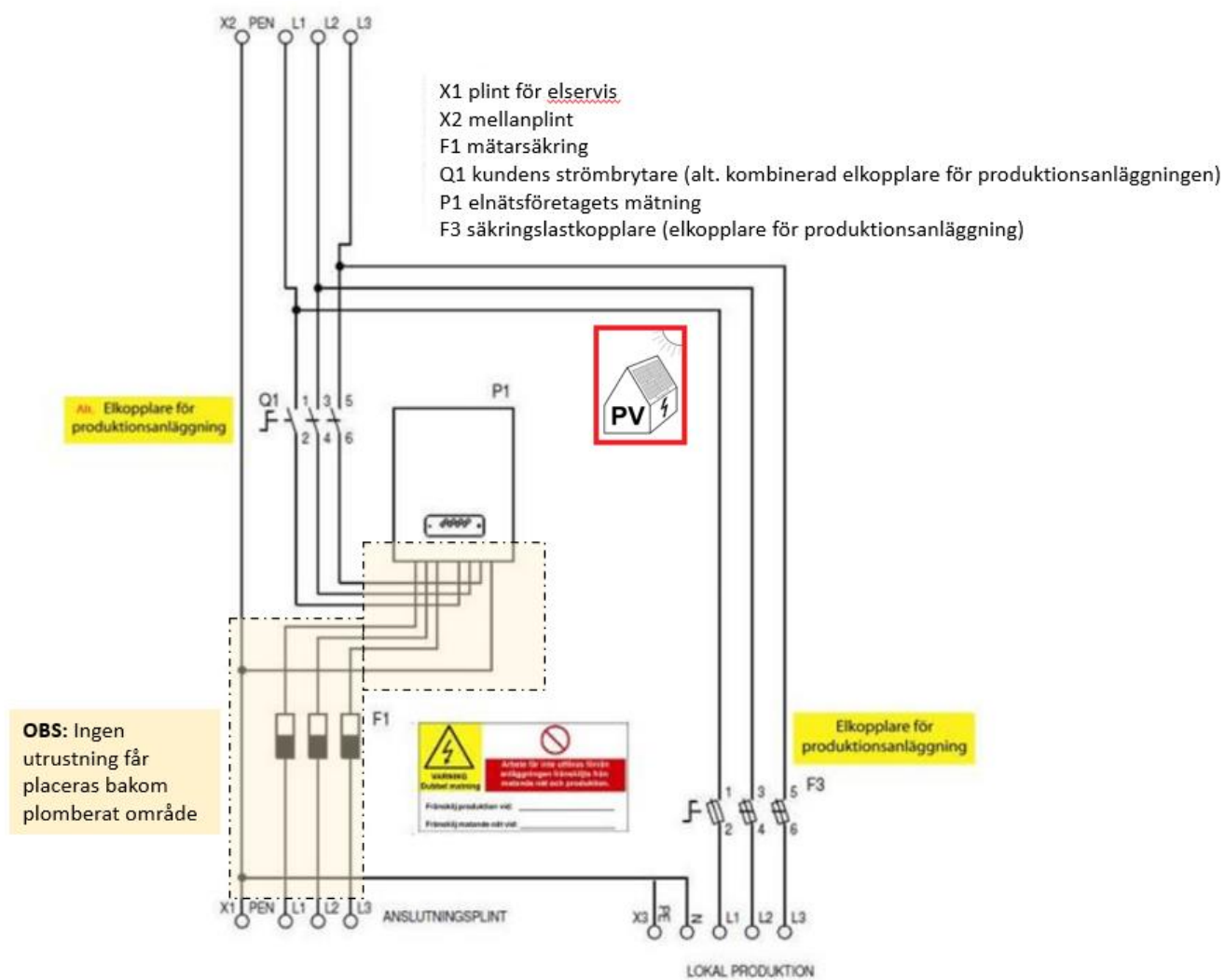
Figur 7 Inkoppling och märkning.
