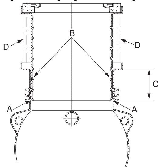
Figur 9. Förlängningsdelens axialläge.
