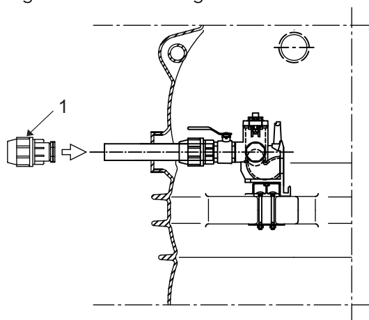
Figur 13. Röranslutning.
