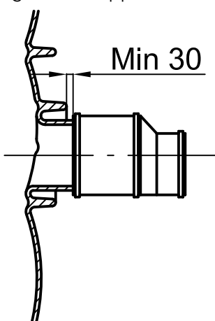
Figur 17. Inloppsrörsmuff.
