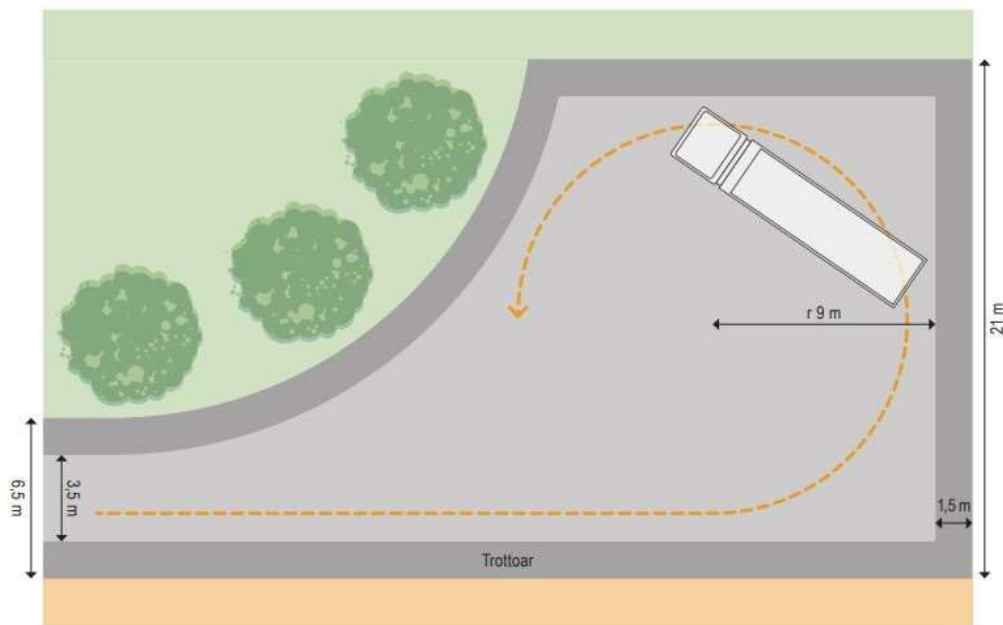
Figur 1 Vändplats för baklastande hämtningsfordon. Utdrag från Avfall Sveriges handbok avfallsutrymmen 2018. Bild: Sara Sundin, Ramboll.
