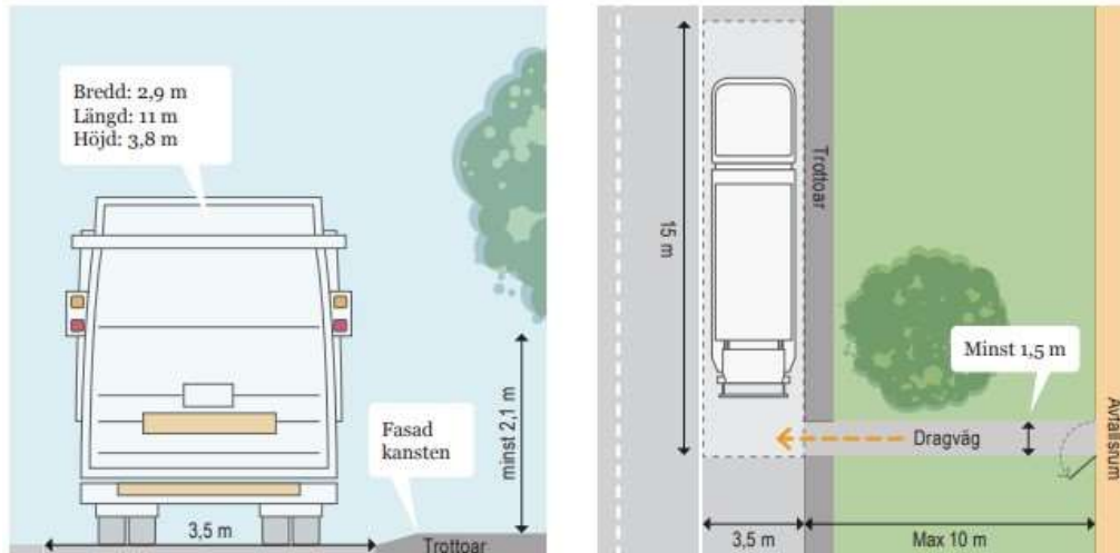
Figur 2 Alternativ vändplats till figur 1 för baklastade hämtningsfordon. Utdrag från Avfall Sveriges handbok avfallsutrymmen 2018. Bild: Sara Sundin, Ramboll.
