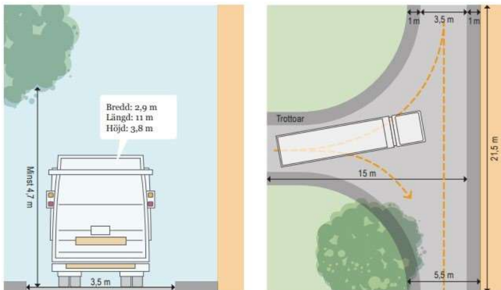
Figur 3 Alternativ vändplats till figur 1 för baklastade hämtningsfordon. Utdrag från Avfall Sveriges handbok avfallsutrymmen 2018. Bild: Sara Sundin, Ramboll.
