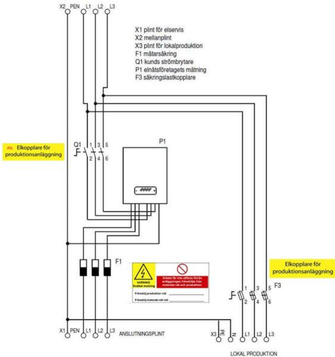
Figur 7 Inkoppling och märkning i mäterskåp
